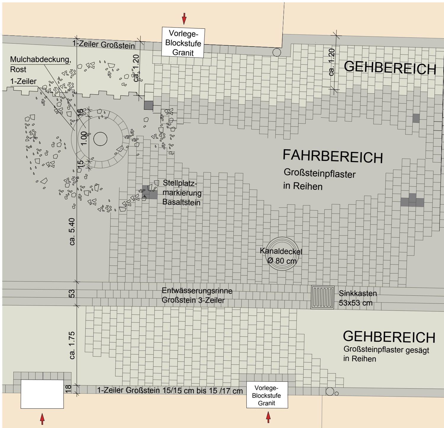
BURGLENGENFELD - NEUGESTALTUNG RATHAUSSTRASSE - DETAILSCHNITT - FUSSWEG BEIDSEITIG M 1:50 - 19.09.2013 UB
